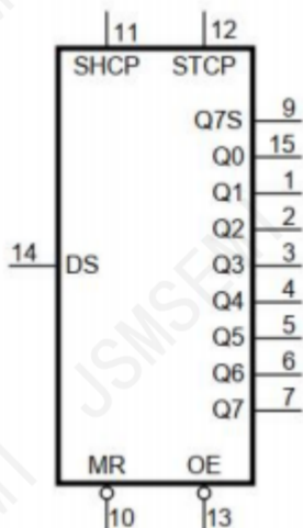
图 1 逻辑符号
