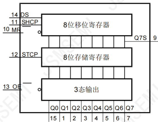
图 4 功能框图
