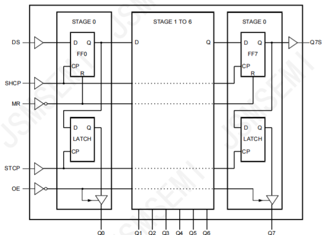
图 3 逻辑框图
