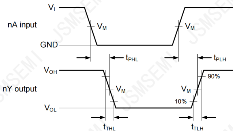
图5 输入 (nA) 到输出 (nY) 传输延迟
