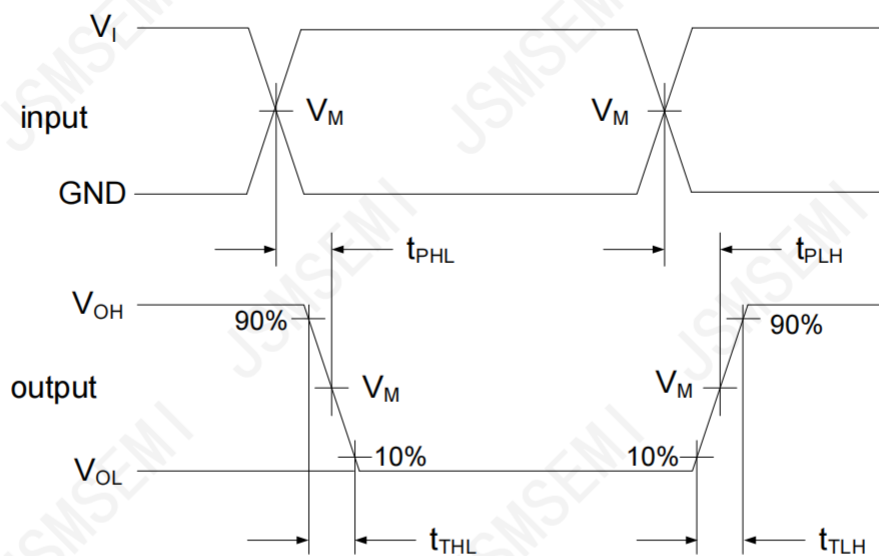
图 3 传输延时，输出转换时间
