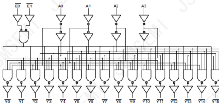
图 1 功能框图
