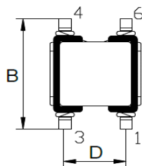
底视图 Bottom view
