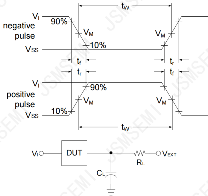
图2 负载线路
