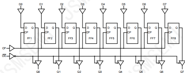
图 3 逻辑框图
