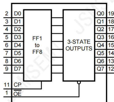
图 4 功能框图
