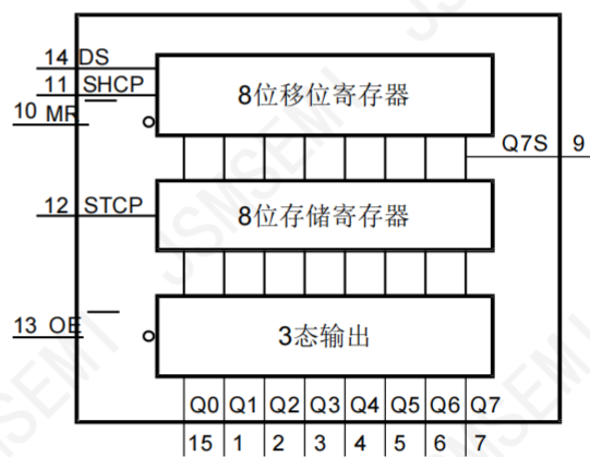
图 4 功能框图
