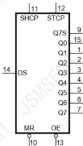
图 1 逻辑符号
