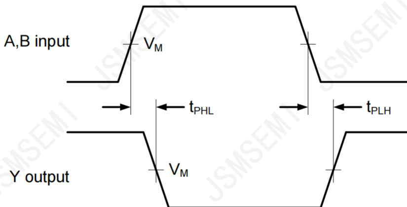
图5 输入（A和B）到输出（Y）传输延迟及输出转换时间
