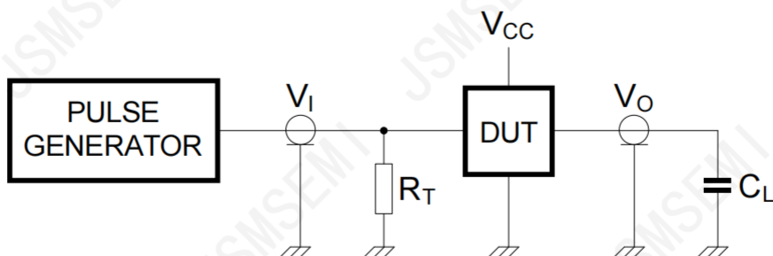
图4 测量开关时间的测试电路
