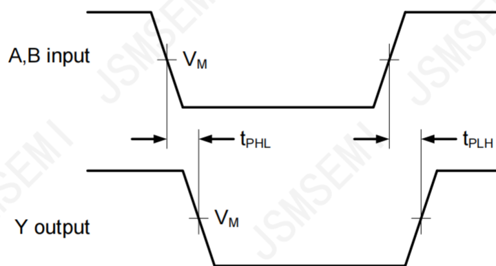
图5 输入（A和B）到输出（Y）的传输延时
