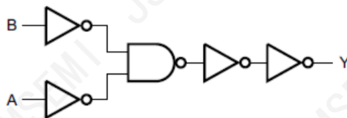
图 2 逻辑框图
