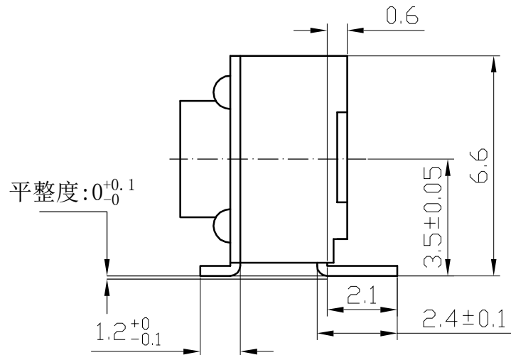
PCB线路板安装图(±0.1)
