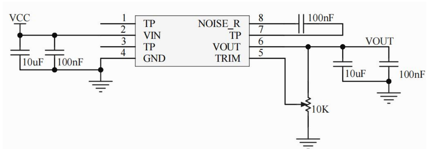
图 5 输出 10V 基准源
