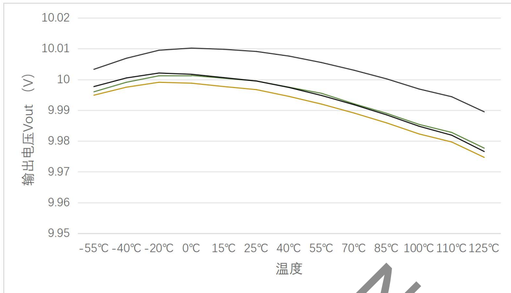
图 4 输出电压 VS 温度曲线图
