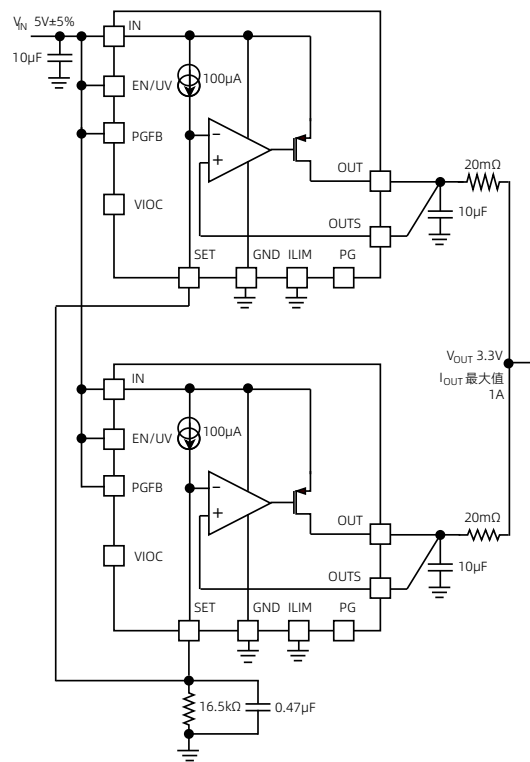
图 31 芯片并联
