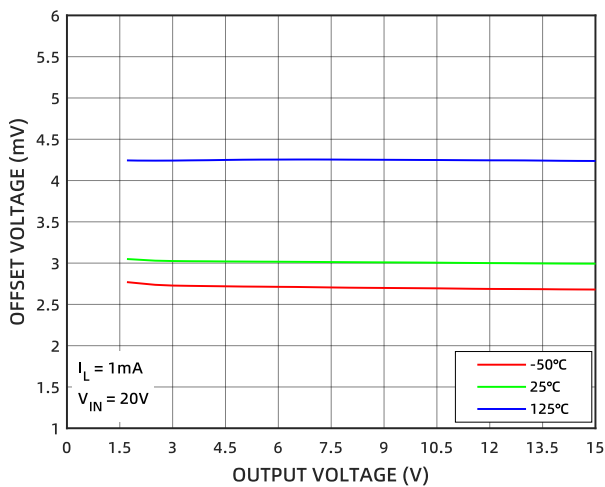
图 5 失调电压随输出电压的变化
