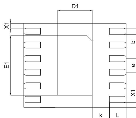
底视图
