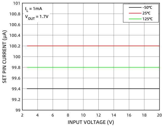
图 3 SET 管脚电流随输入电压的变化
