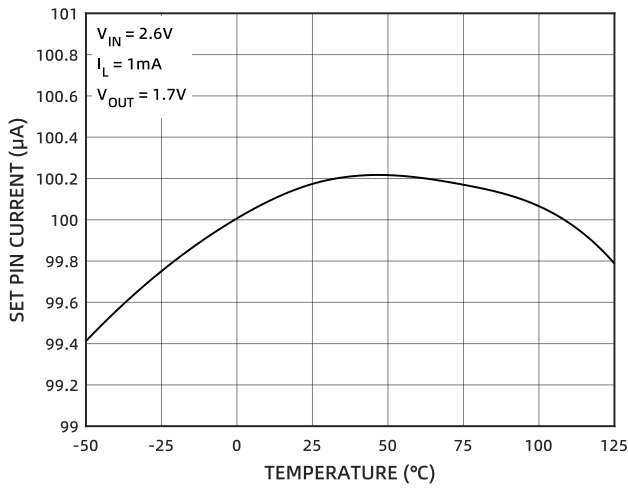
图 1 SET 管脚电流的温度特性
