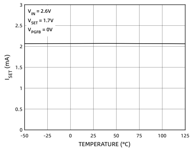
图 16 快速启动期间 I_{SET} 的温度特性
