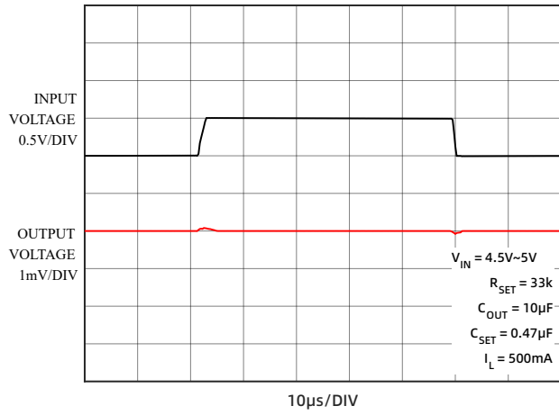
图 25 线性瞬态响应
