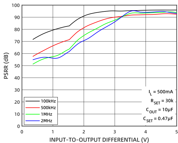
图 21 PSRR (不同压差下)
