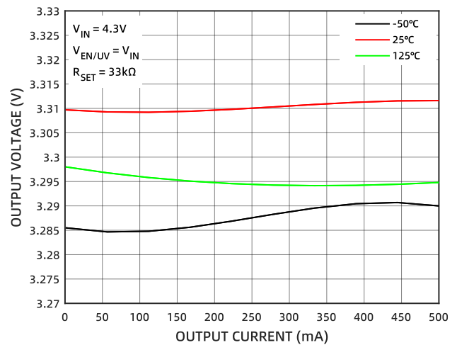
图 6 负载调整率
