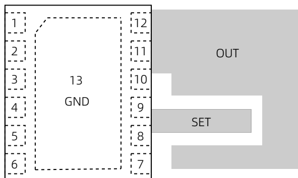
图 29 保护环布局
