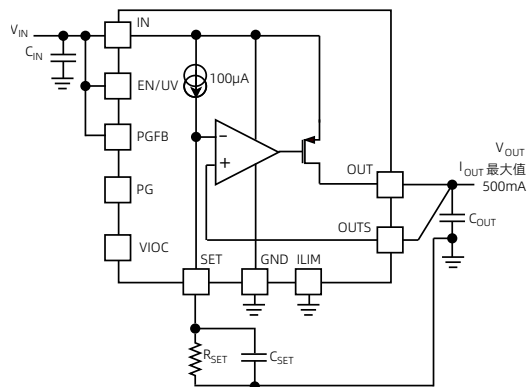
图 30 C OUT 和 C SET 连接实现稳定性
