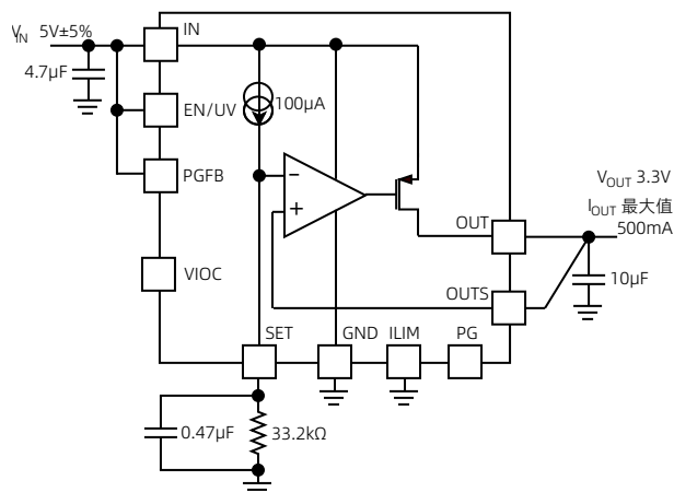
图 28 可调稳压器的典型应用
