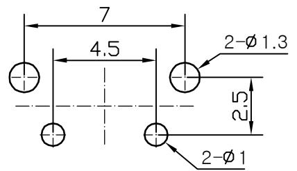
PCB线路板安装图(±0.1)
