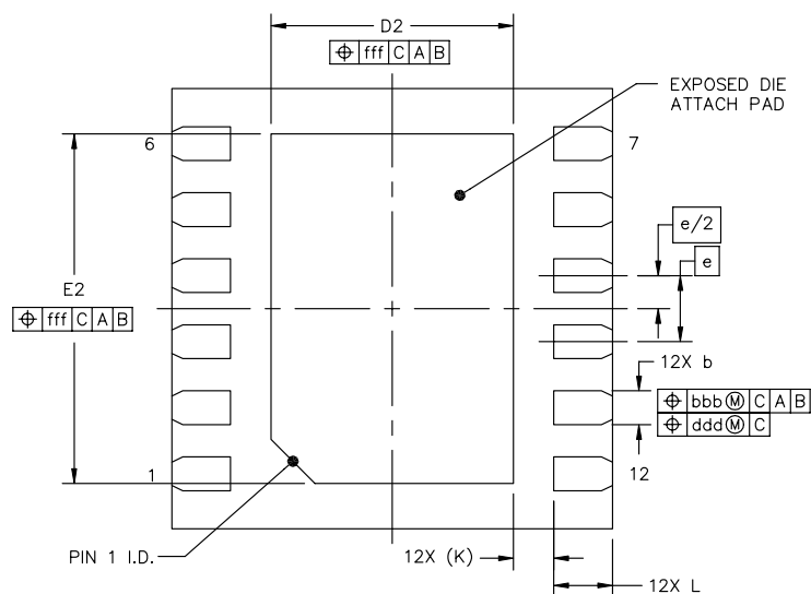
底视图
