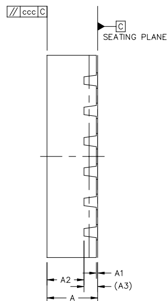
侧视图
