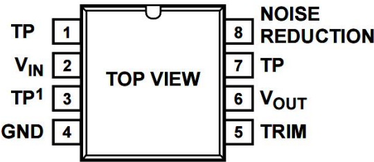
图 2 引脚排列图（顶视图）
