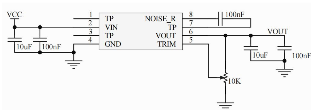
图 5 输出 5V 基准源
