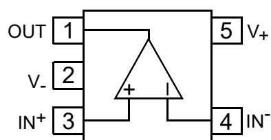
SOT-23-5L
