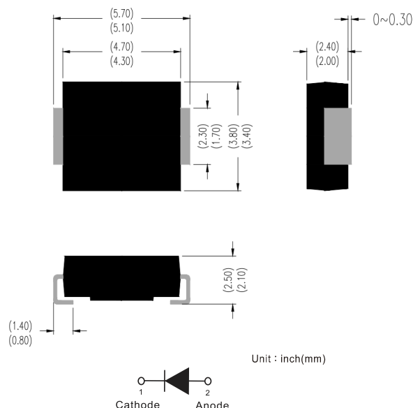
DO214-AA (SMB)
