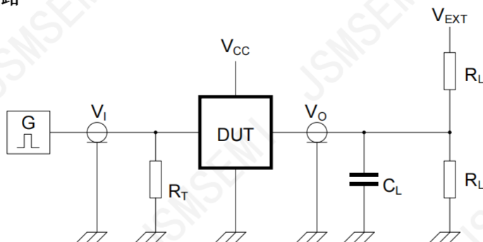
图4 测试开关时间的测试电路
