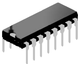
DIP-16-300-2.54
