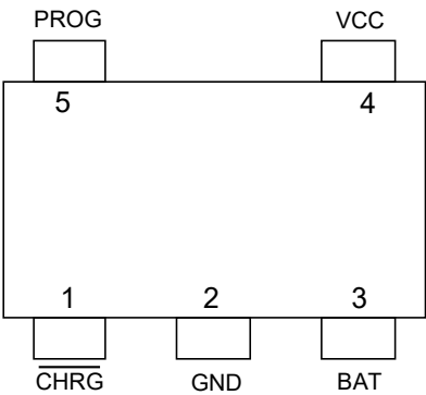
SOT23-5
