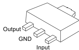
SOT-89
