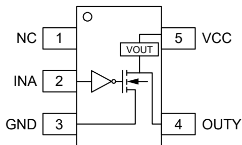
SOT23-5/SC70-5
