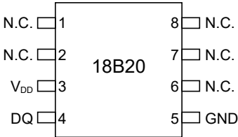
SOP8
