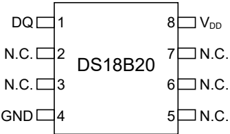
MSOP8
