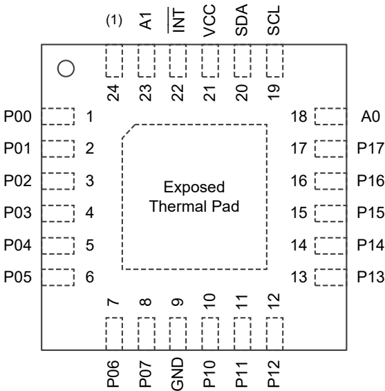
VQFN-24-EP(4x4)
