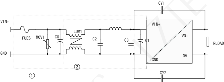
图中第①部分用于 EMC 测试；第②部分用于 EMI 滤波，可依据需求选择
