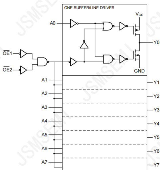
图 4 逻辑框图
