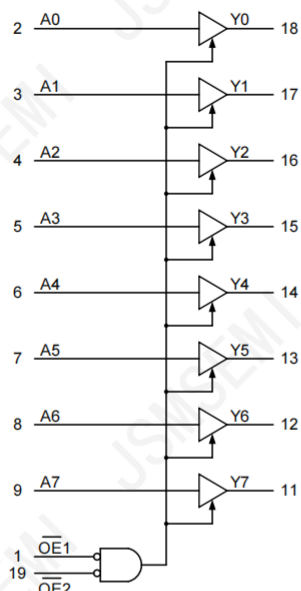
图 1 逻辑符号
