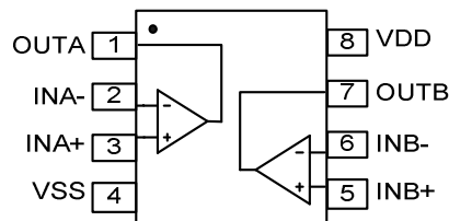
SOP-8 TSSOP-8
