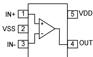
SOT23-5 SC70-5
