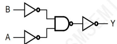
图 3 逻辑框图
