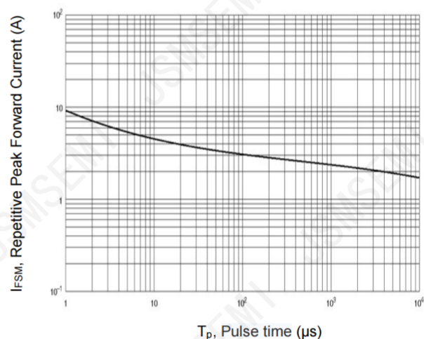
Fig 4. I_{FSM} vs. T_p
