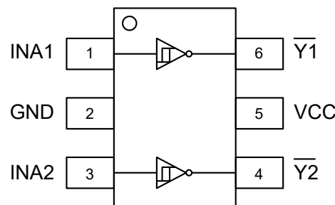
SOT23-6/SC70-6
