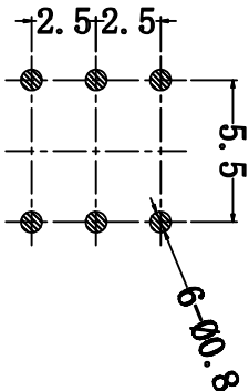
PCB参考图
