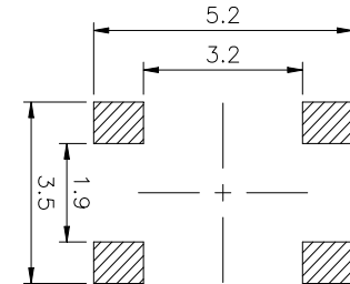
PCB. 焊接图
