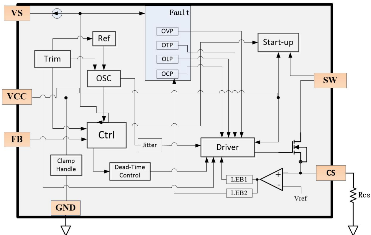
■ 电路结构框图
