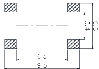
PCB. 焊接图
