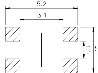
PCB. 焊接图
