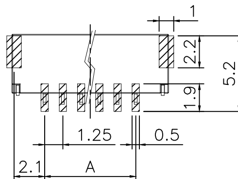
PCB. 焊接图
