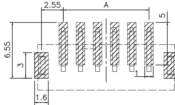
PCB. 焊接图
