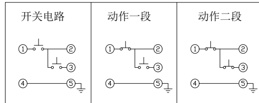
电路图
