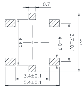
PCB. 焊接图
