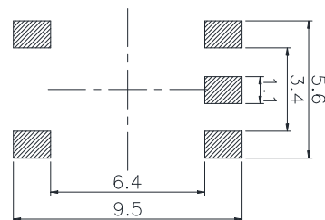
PCB. 焊接图
