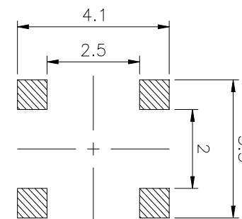
PCB. 焊接图
