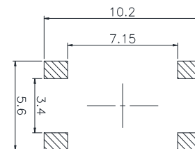
PCB. 焊接图
