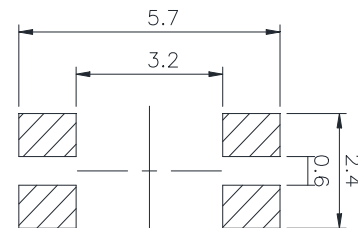
PCB. 焊接图
