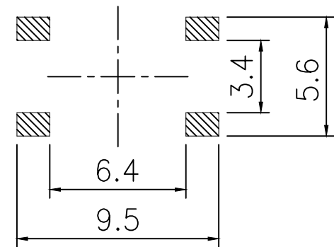
PCB. 焊接图
