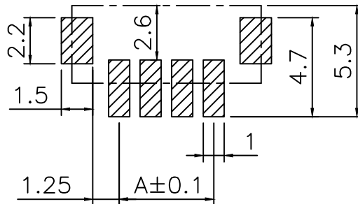
PCB. 焊接图
