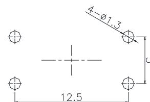
PCB. 焊接图
