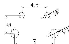
PCB. 焊接图
