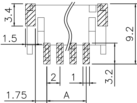
PCB. 焊接图
