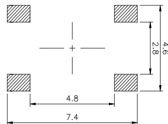
PCB. 焊接图
